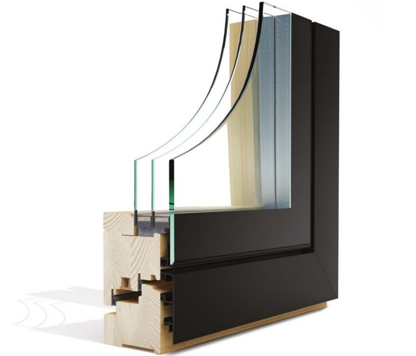
VIZIJA XL U_g 0,5 U_w 0,80
